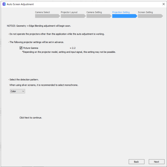
设定初始化确认界面 (几何矫正和边缘混合：未执行黑电平矫正时)
