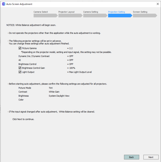
设定初始化确认屏幕 (白平衡调整)
