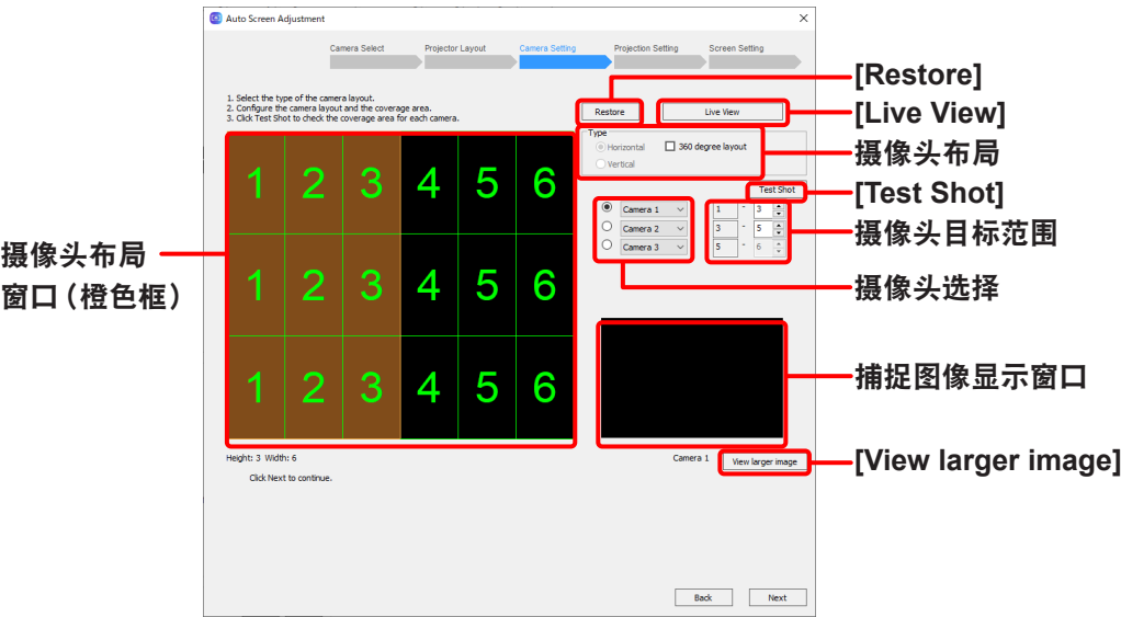
摄像机布局界面
